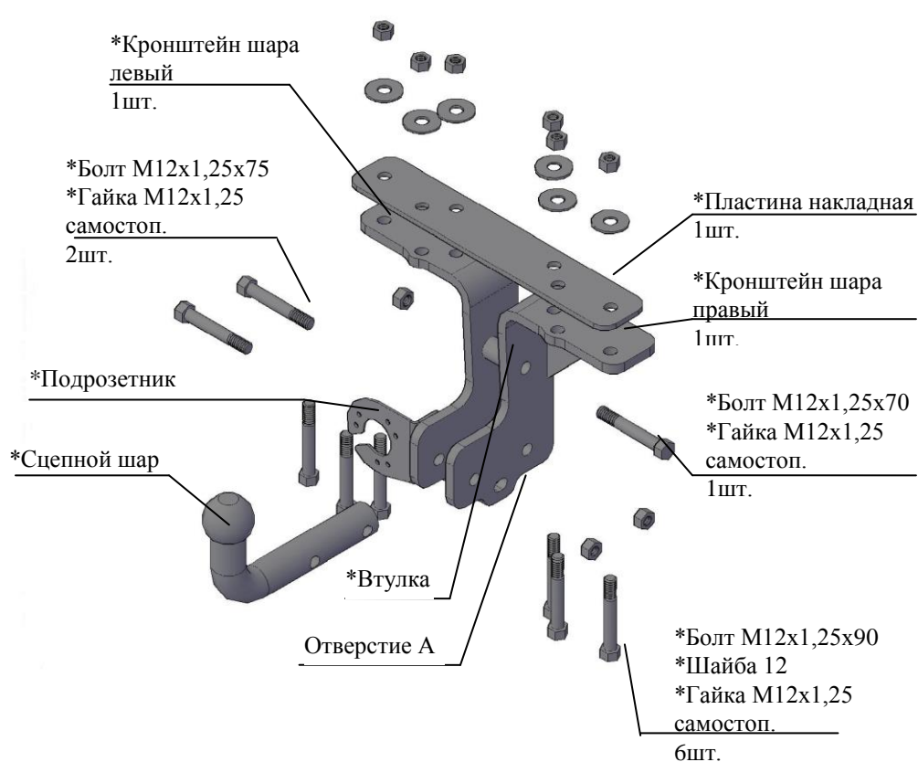
Рис.1 Тягово-сцепное устройство 7760
