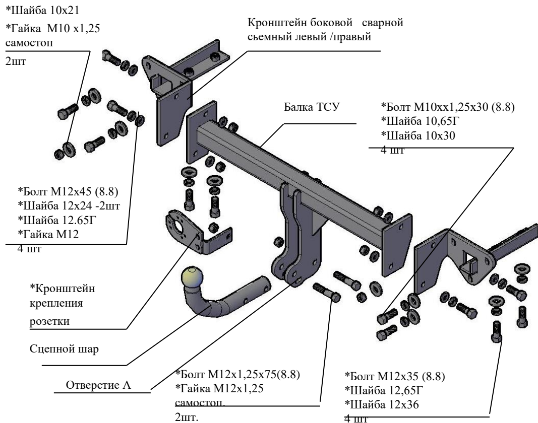
Рис.1 Тягово-сцепное устройство 8510 .
